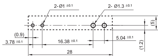
水平安装型
