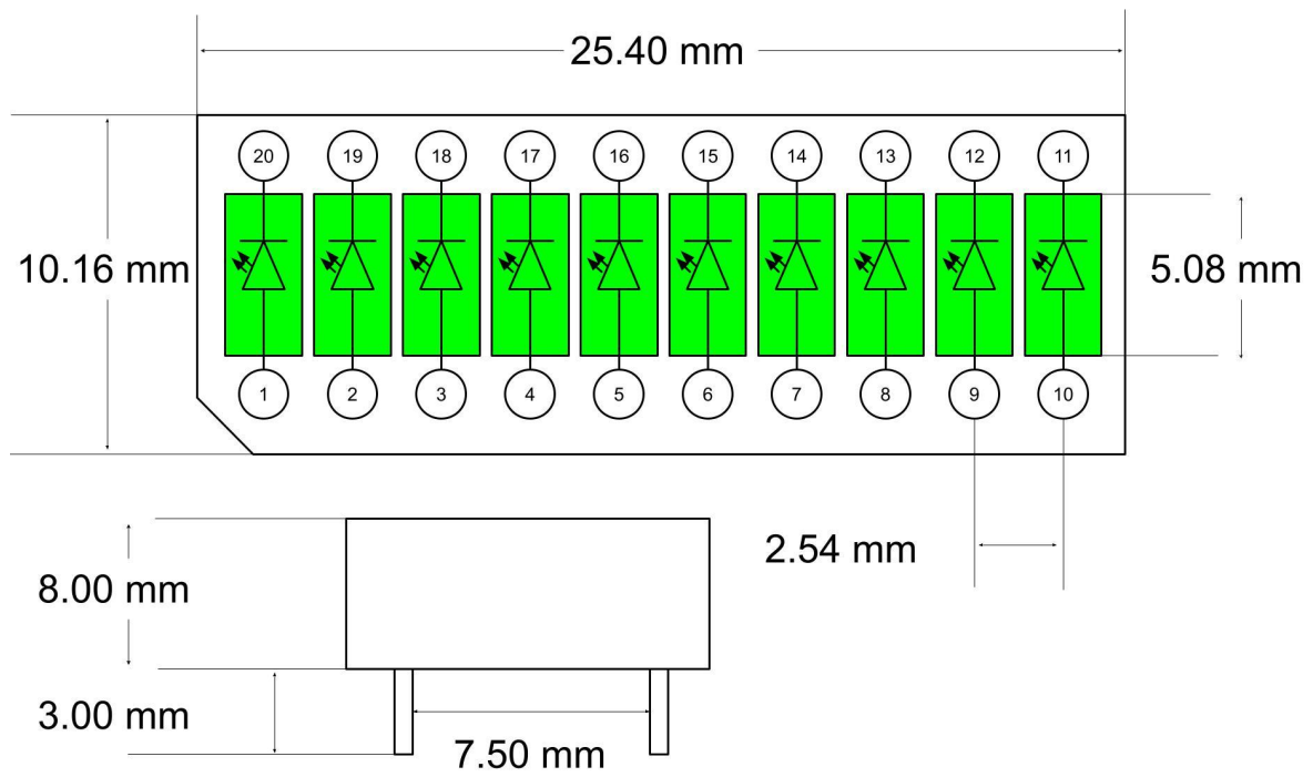
Imagen 2. Dimensiones de una barra de 10 leds.
